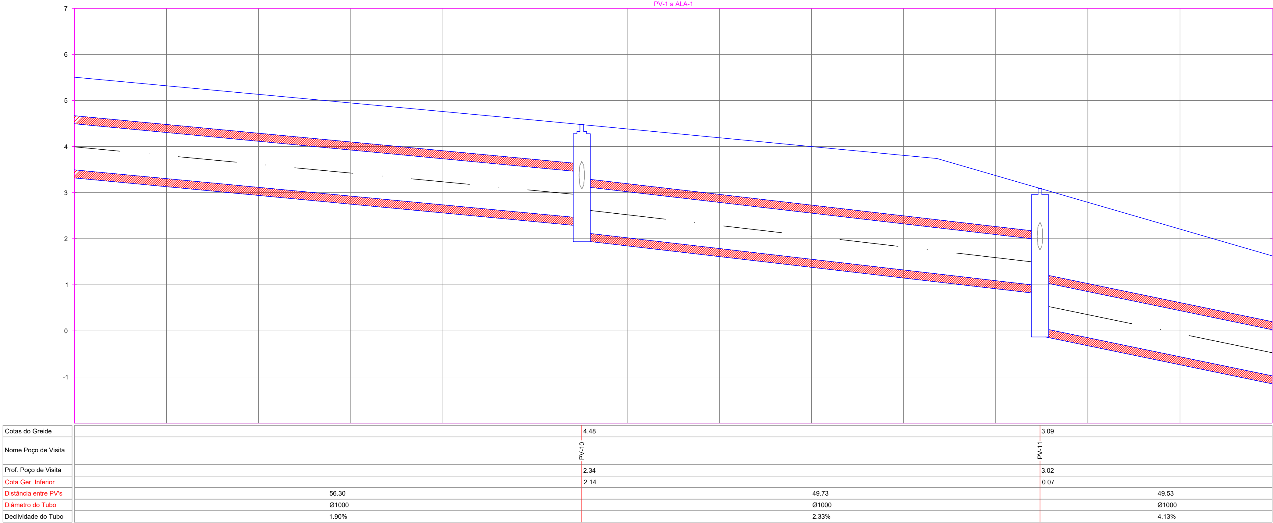
PERFÍL LONGITUDINAL
