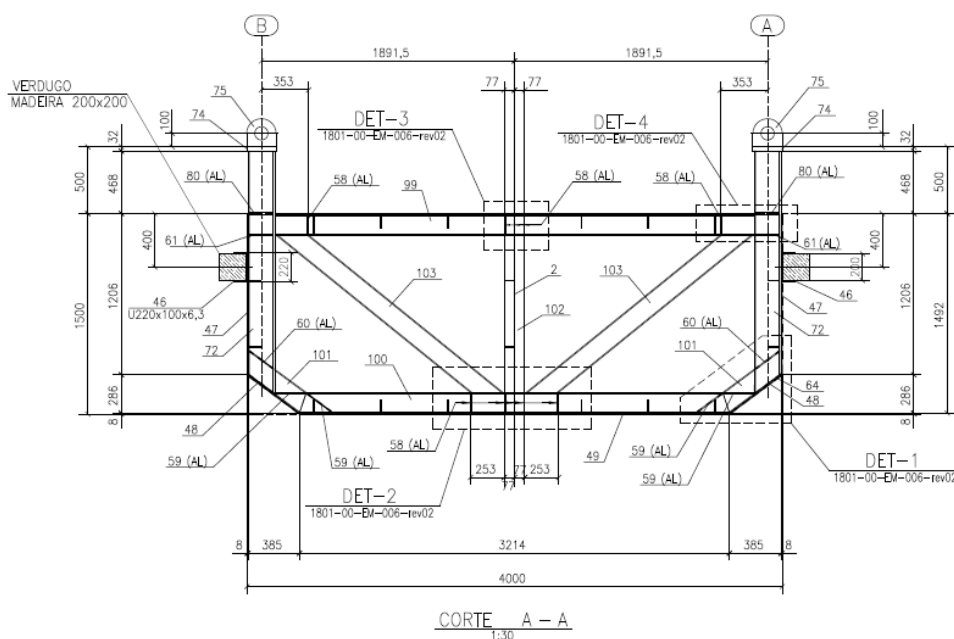
FIGURA 13 – FLUTUANTES – SEÇÃO TRANSVERSAL ENRIJECEIDA
