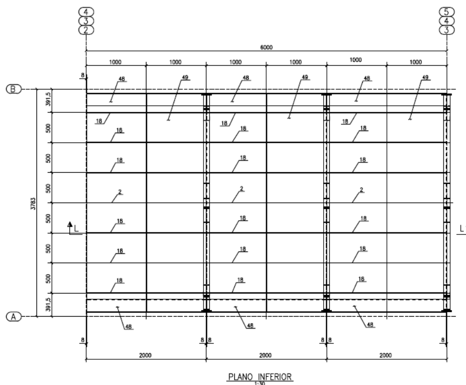
FIGURA 12 – FLUTUANTES – PLANTA INFERIOR
