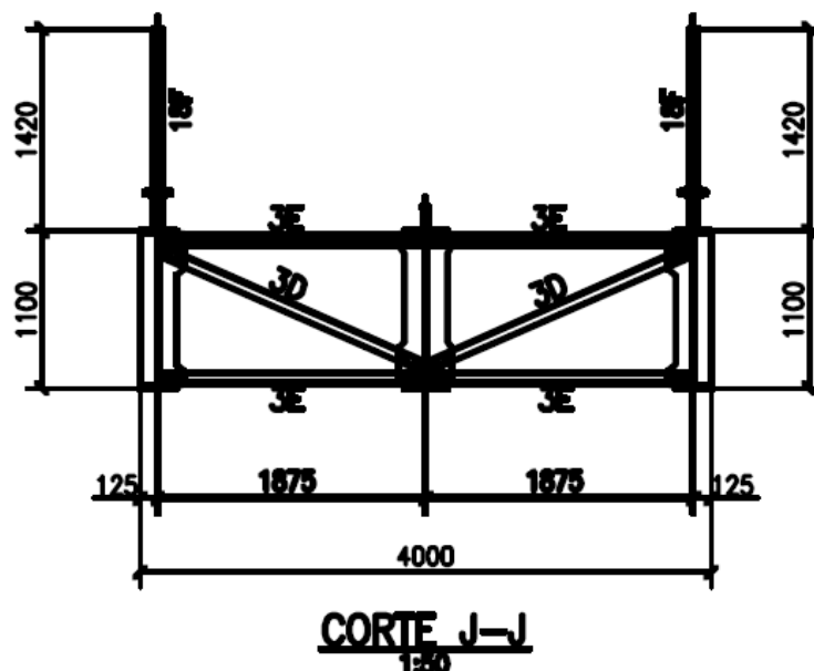
FIGURA 6 – PASSARELA FIXA – VIGAMENTO METÁLICO – SEÇÃO TRANSVERSAL
