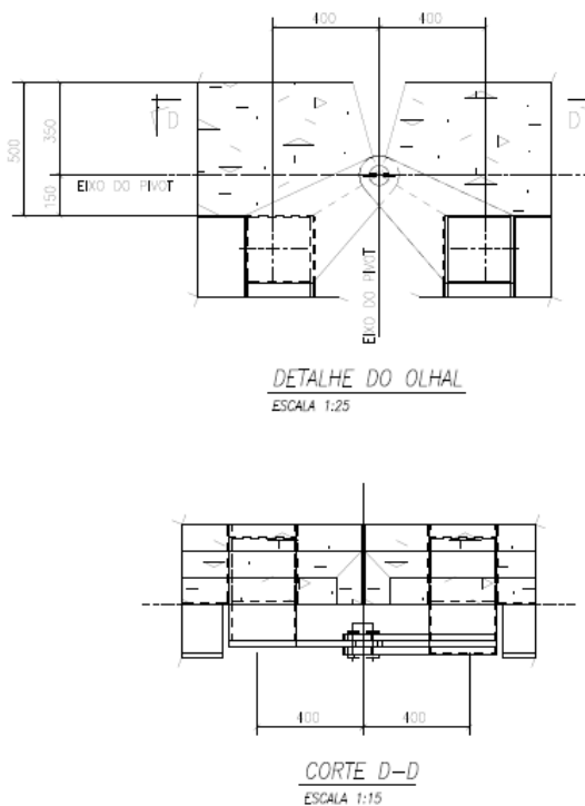
FIGURA 20 – FLUTUANTES – OLHAIS E PINOS
