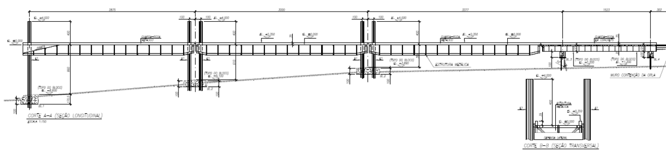
FIGURA 1 – PERFIL LONGITUDINAL DO PÍER PADRÃO
