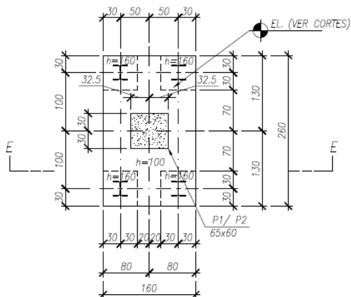
BLOCOS BL.1 (6x) e BL.2 (6x) – PLANTA VÁLIDO PARA SEÇÕES 1 a 6 ESCALA 1:50 (160x260/100)
