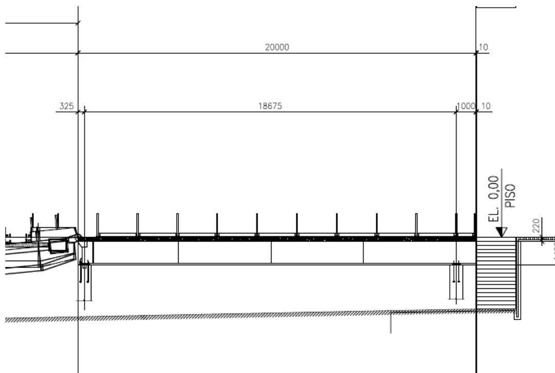
FIGURA 4 – PASSARELA FIXA – ELEVACÃO
