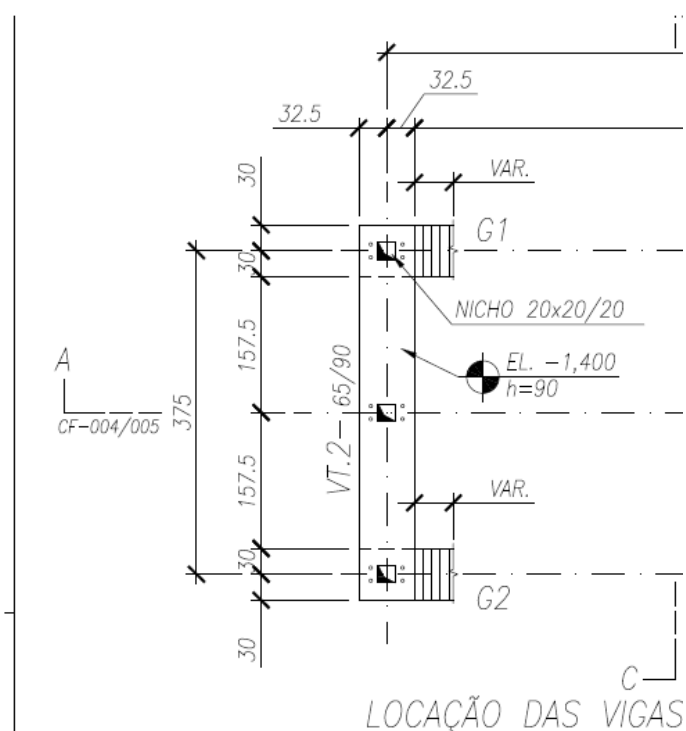
FIGURA 9 – PASSARELA FIXA – TRAVESSA DE APOIO
