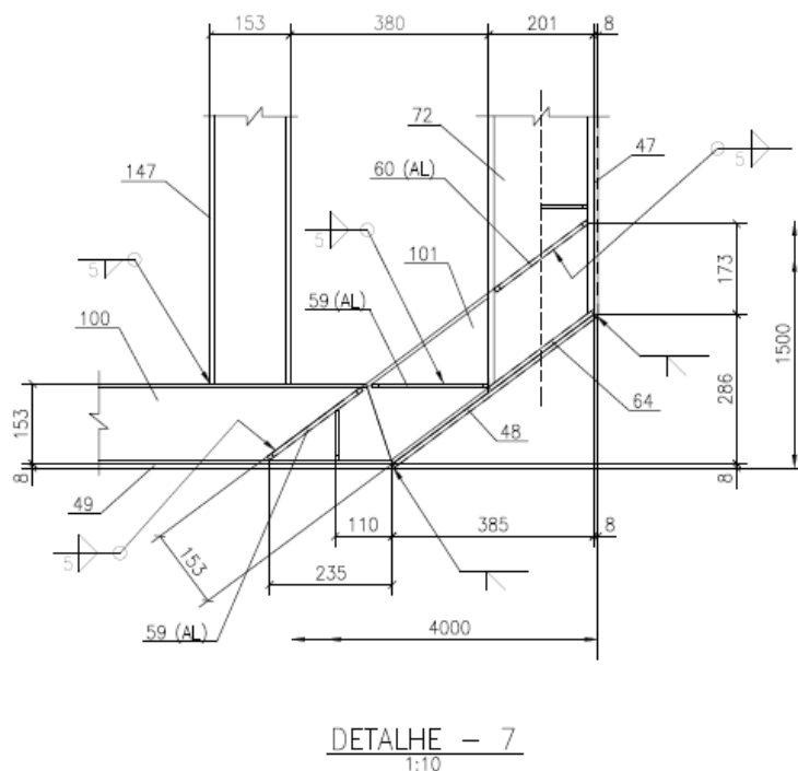
FIGURA 17 – FLUTUANTES – ENCONTRO DOS PERFIS
