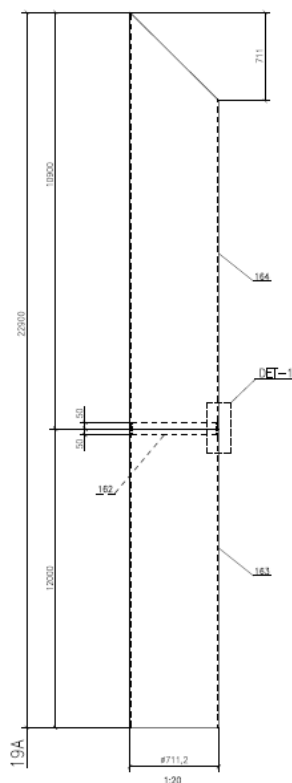
FIGURA 19 – FLUTUANTES – PÓRTICOS / ESTACAS / PILARES
