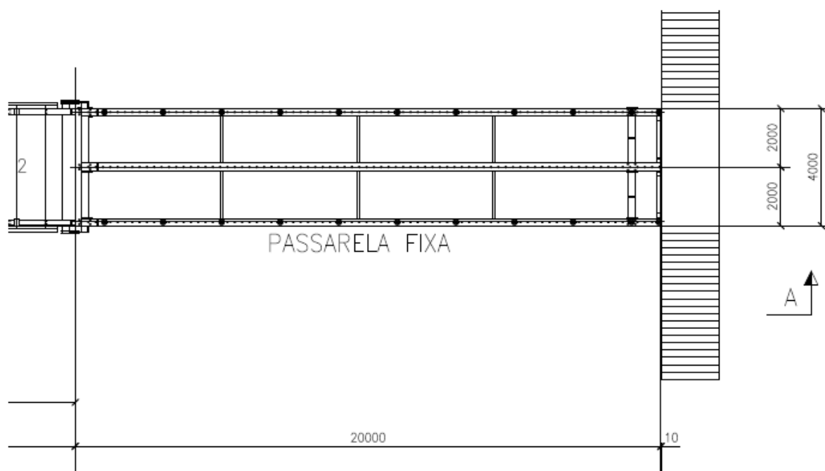
FIGURA 3 – PASSARELA FIXA - PLANTA
