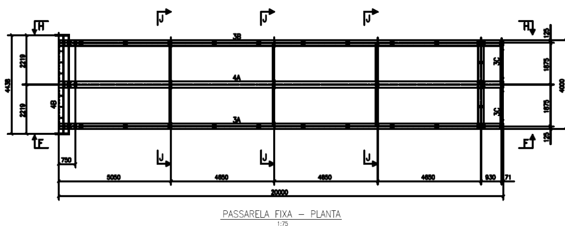
FIGURA 5 – PASSARELA FIXA – VIGAMENTO METÁLICO - PLANTA
