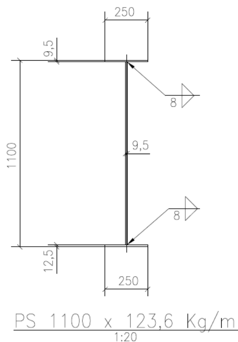
FIGURA 8 – PASSARELA FIXA – VIGAMENTO PRINCIPAL
