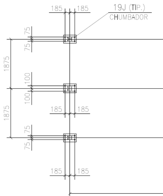
FIGURA 7 – PASSARELA FIXA – CHUMBADORES DE FIXAÇÃO DAS VIGAS
