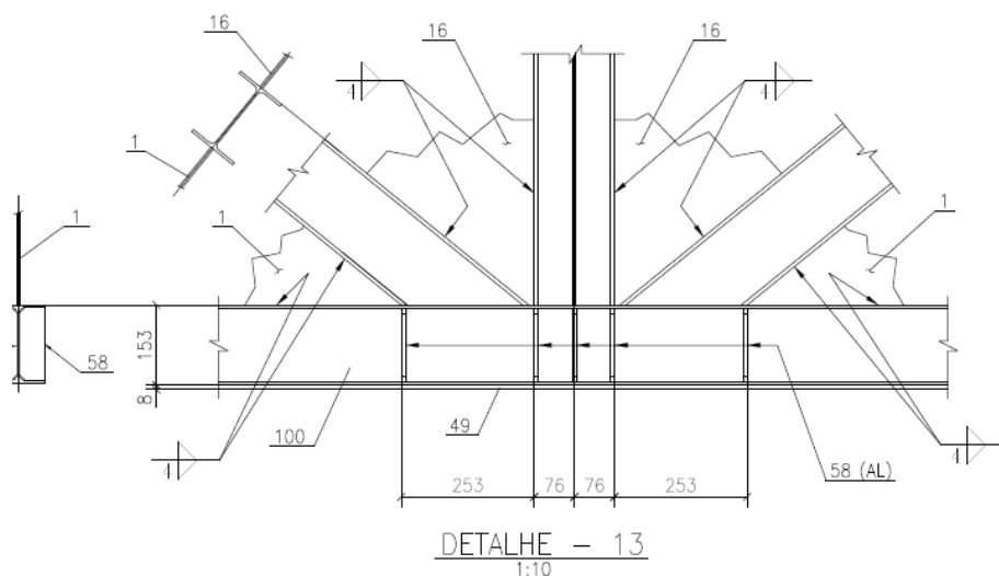
FIGURA 16 – FLUTUANTES – ENCONTRO DOS PERFIS
