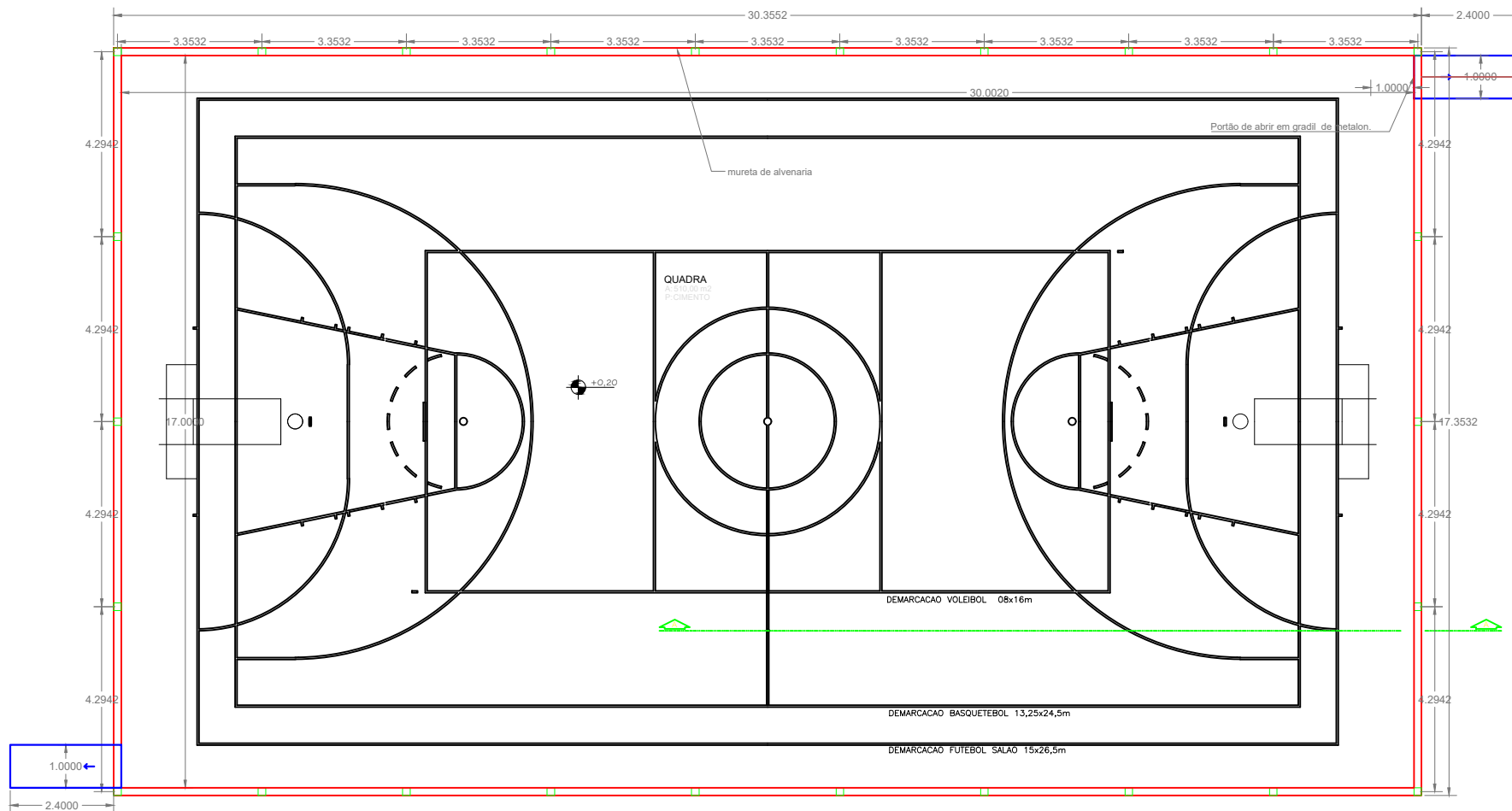
PLANTA BAIXA ESC. 1/150
