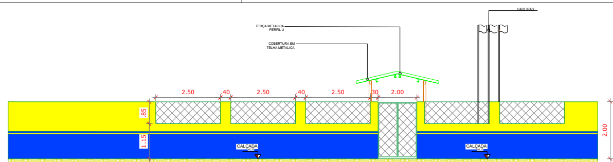
FACHADA DE MURO Escala 1: 100
