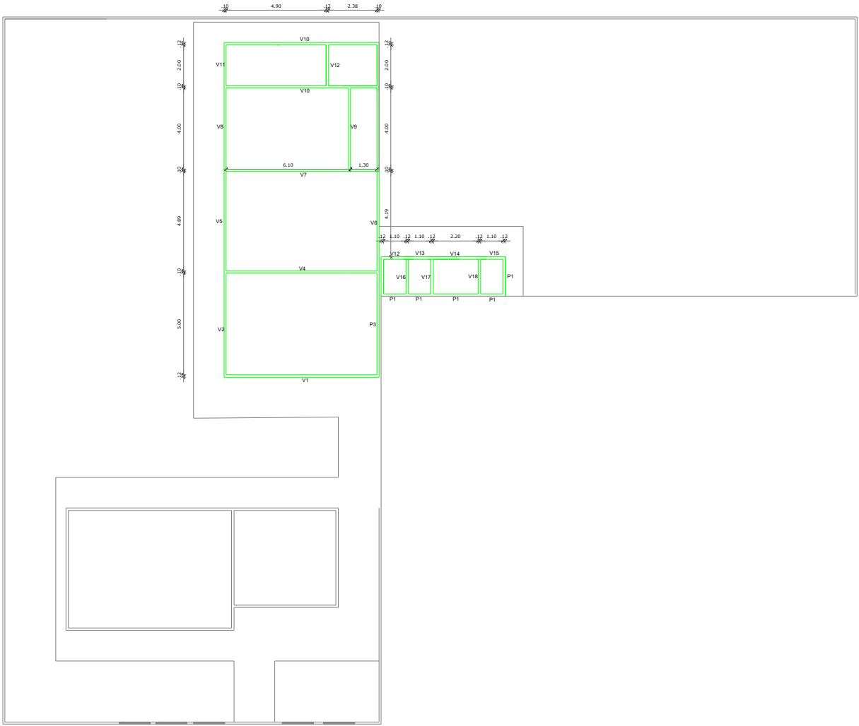
PROJETO ESTRUTURAL - VIGAMENTO ESCOLA SANTA BRÍGIDA COMUNIDADE IGARAPÉ DO PIMENTA - PLANALTO COORDENADAS: (-2.561961, -54.763616) Escala 1 : 75
