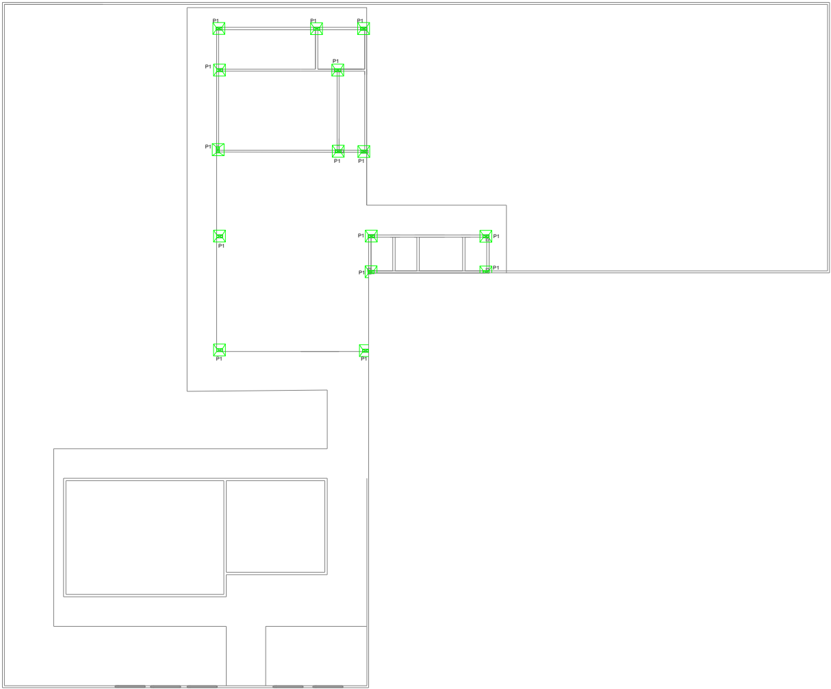
PROJETO ESTRUTURAL - PILARES ESCOLA SANTA BRÍGIDA COMUNIDADE IGARAPÉ DO PIMENTA - PLANALTO COORDENADAS: (-2.561961, -54.763616) Escala 1 : 75
