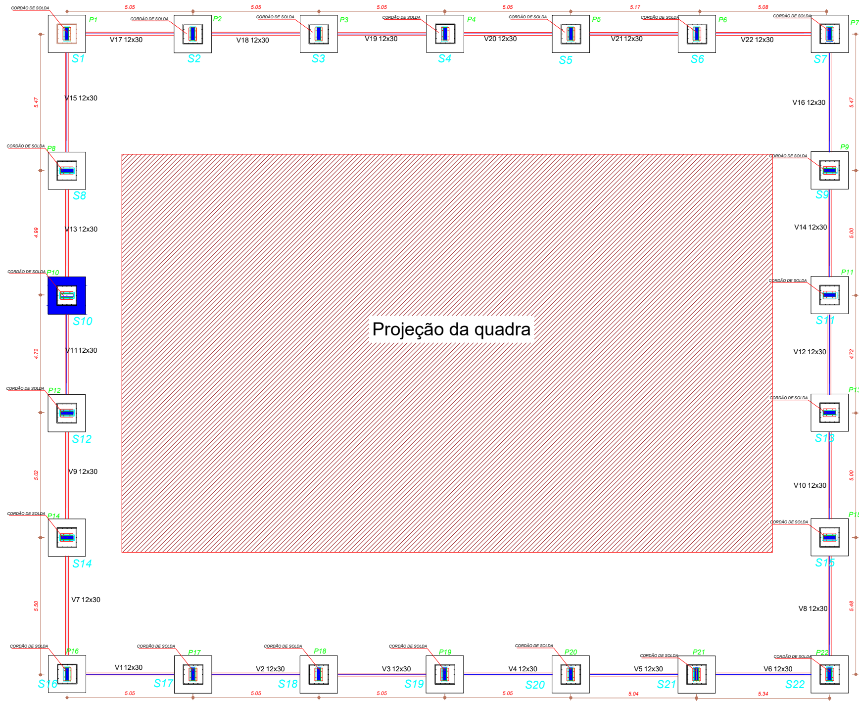
PLANTA DOS BLOCOS E EIXOS DE BALDRAME ESCALA: 1/150
