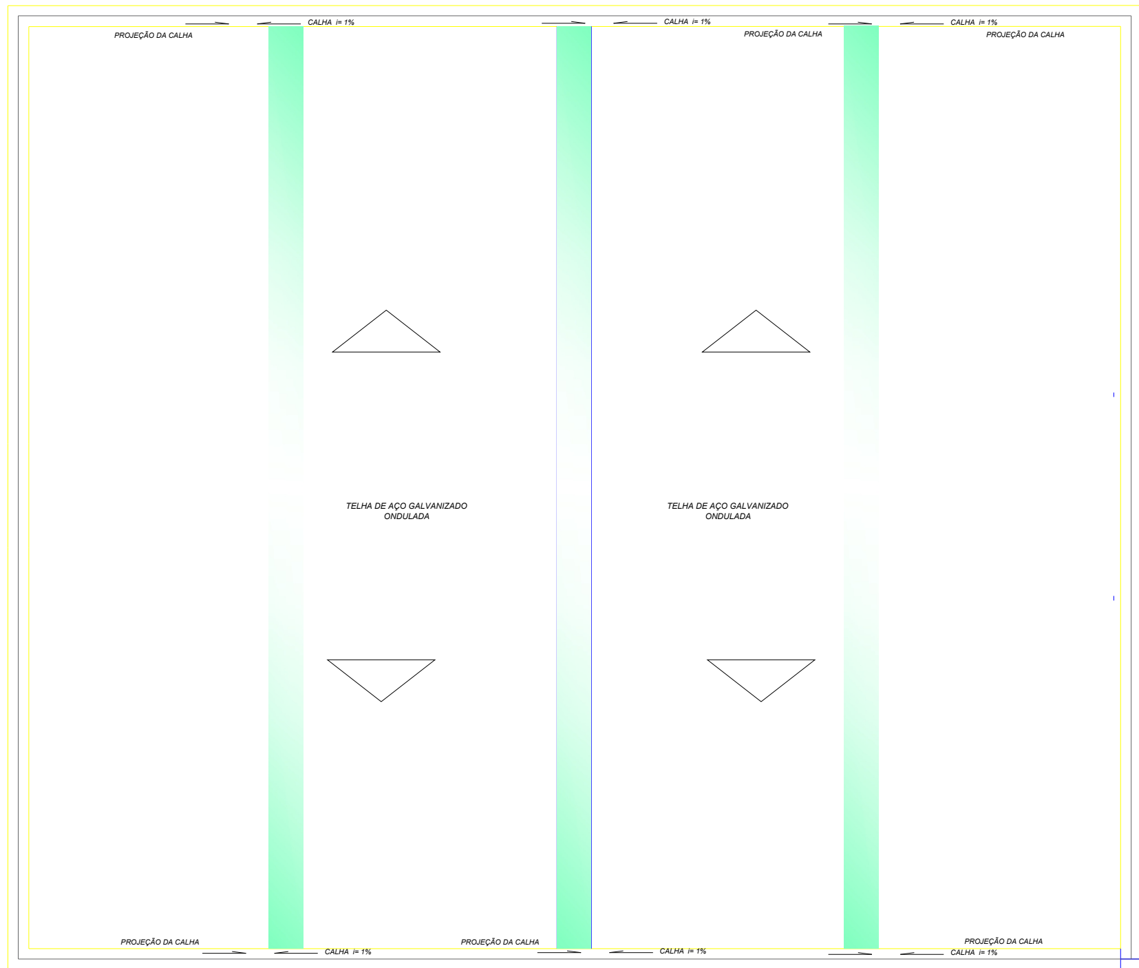
PLANTA DE COBERTURA- QUADRA COBERTA Escala 1: 150
