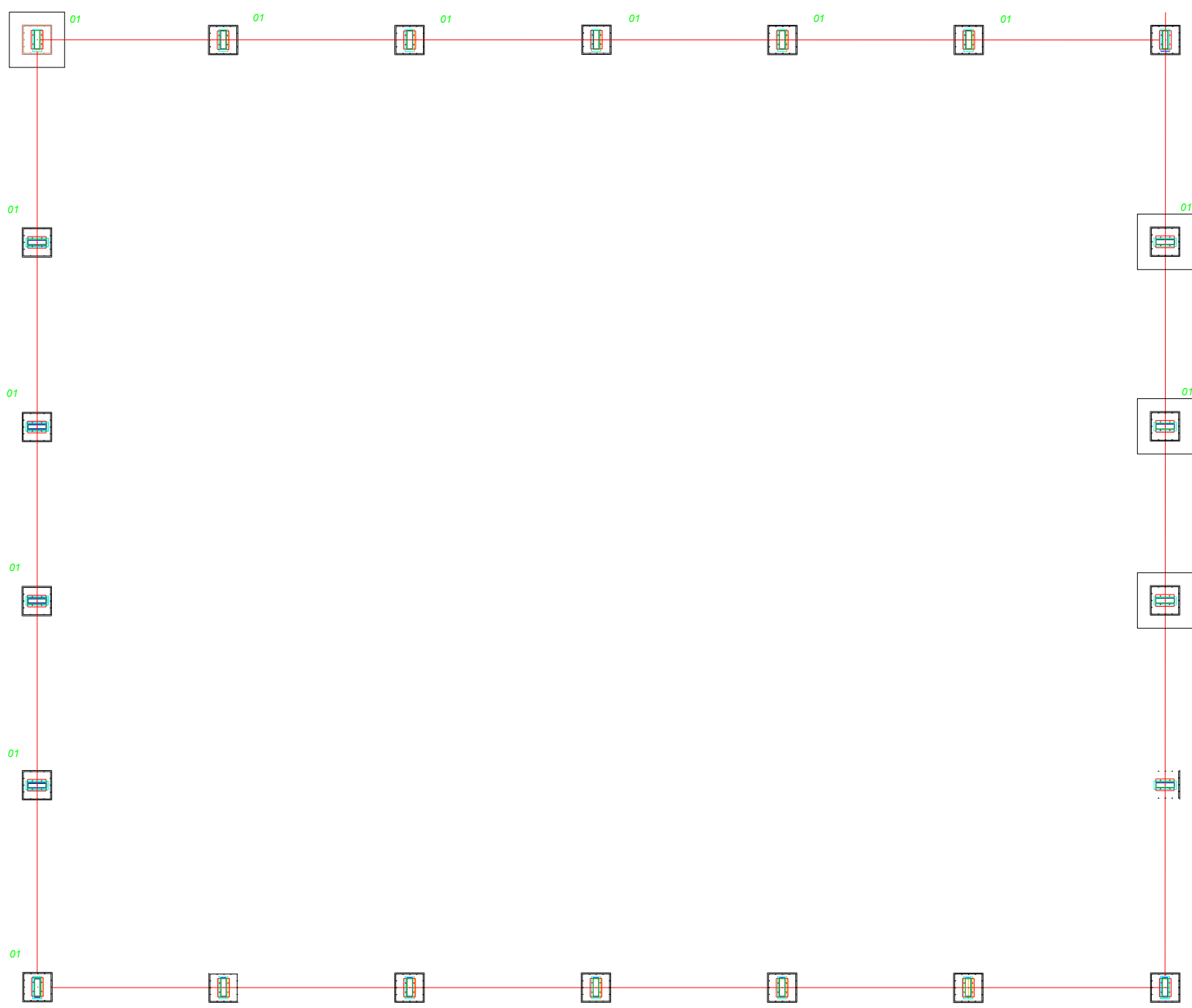
PLANTA DOS BLOCOS E EIXOS DE BALDRAME ESCALA: 1/150
