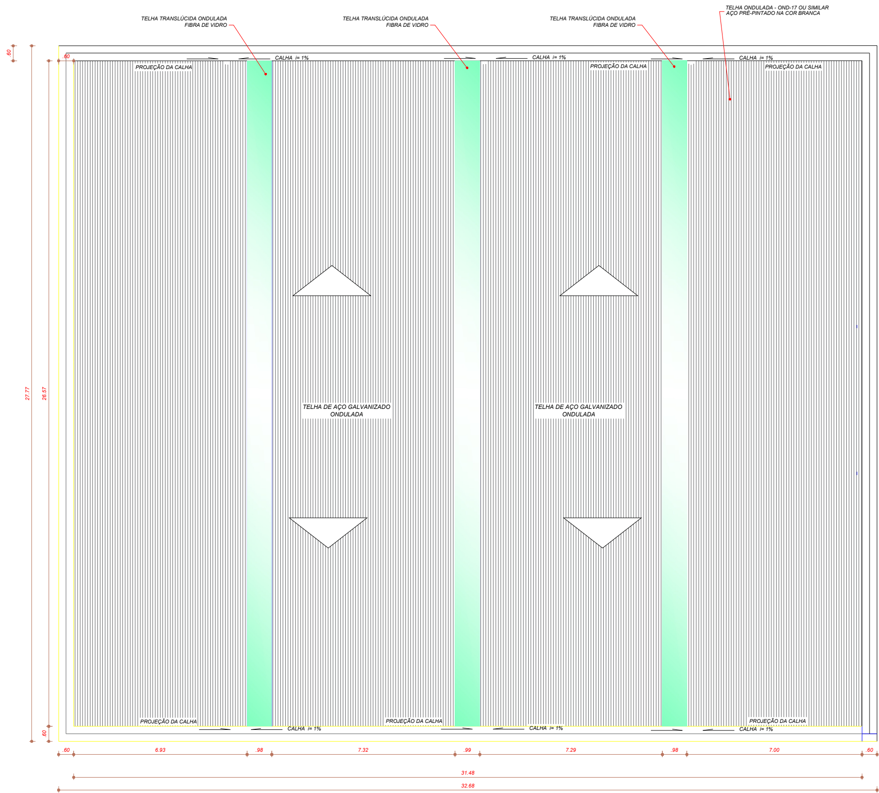
PLANTA DE COBERTURA- QUADRA COBERTA Escala 1: 150
