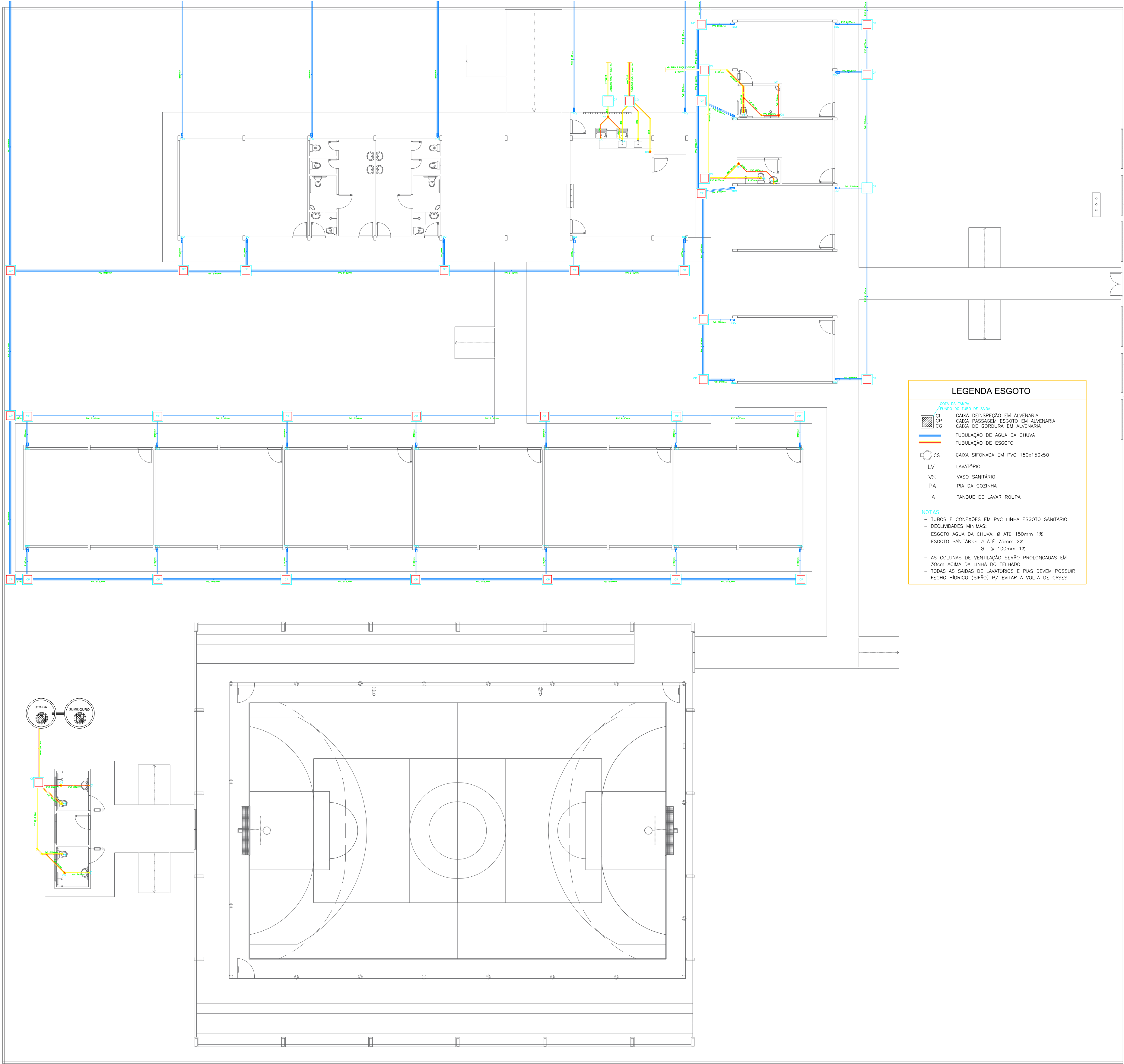
PLANTA DE ESGOTO E AGUA PLUVIAL ESCOLA SÃO PEDRO COMUNIDADE DE BOM JARDIM COORDENADAS: -2.559886, -54.594701 Escala 1 : 150
