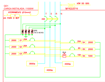
11 DIAGRAMA MULTIFILAR - QD1
