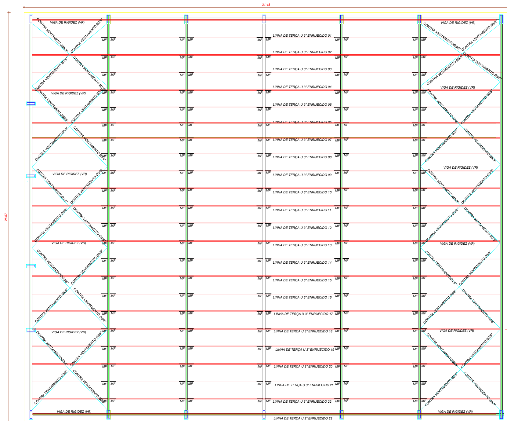
ESTRUTURA DE TELHADO - QUADRA COBERTA Escala 1: 150
