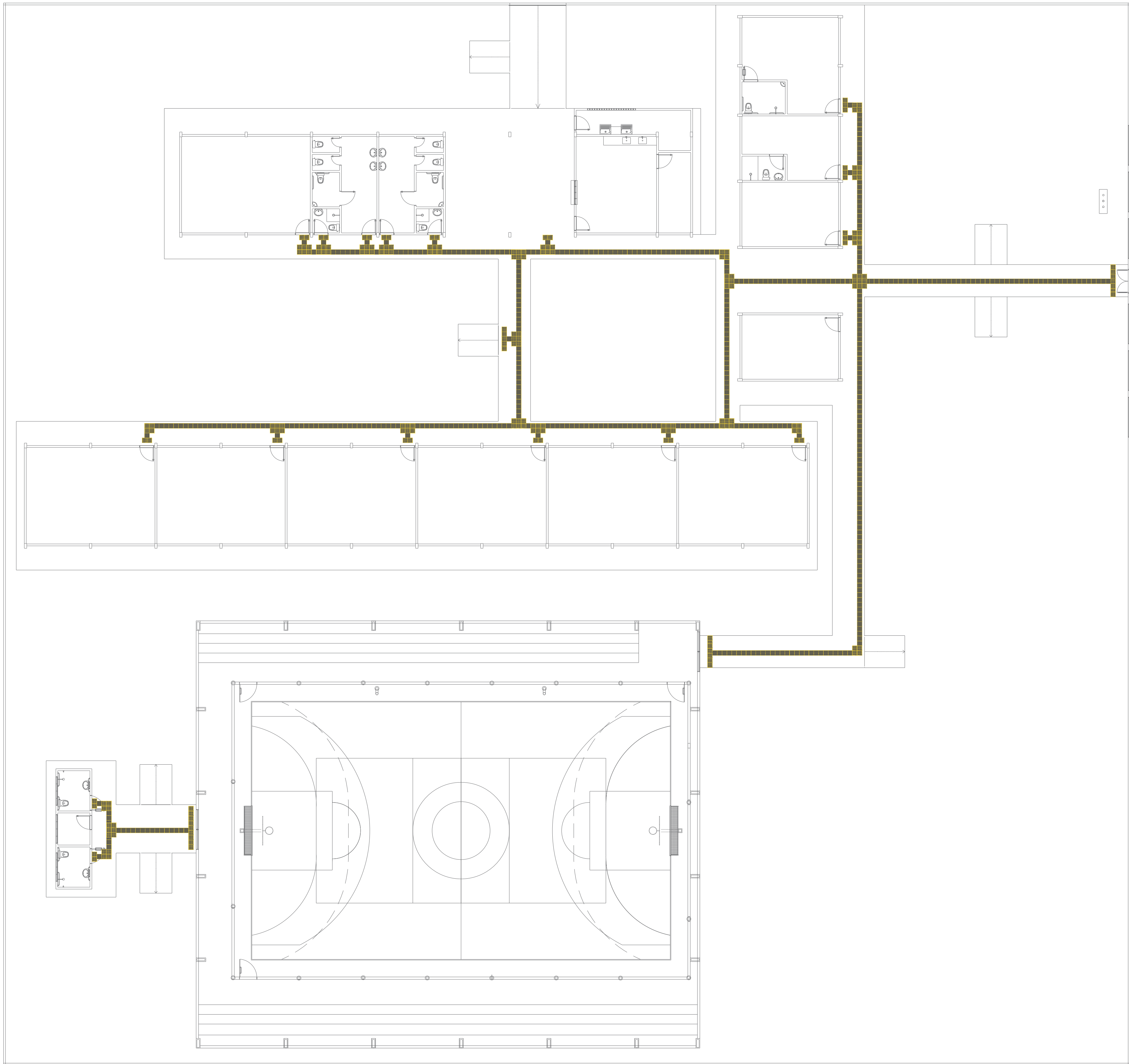
PLANTA BAIXADE PISO TATIL ESCOLA SÃO PEDRO COMUNIDADE DE BOM JARDIM COORDENADAS: -2.559886, -54.594701 Escala 1 : 150
