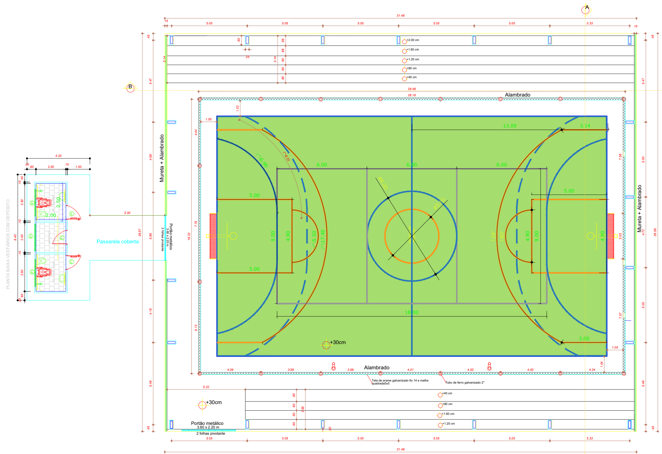
PLANTA BAIXA- QUADRA COBERTA Escala 1: 150
