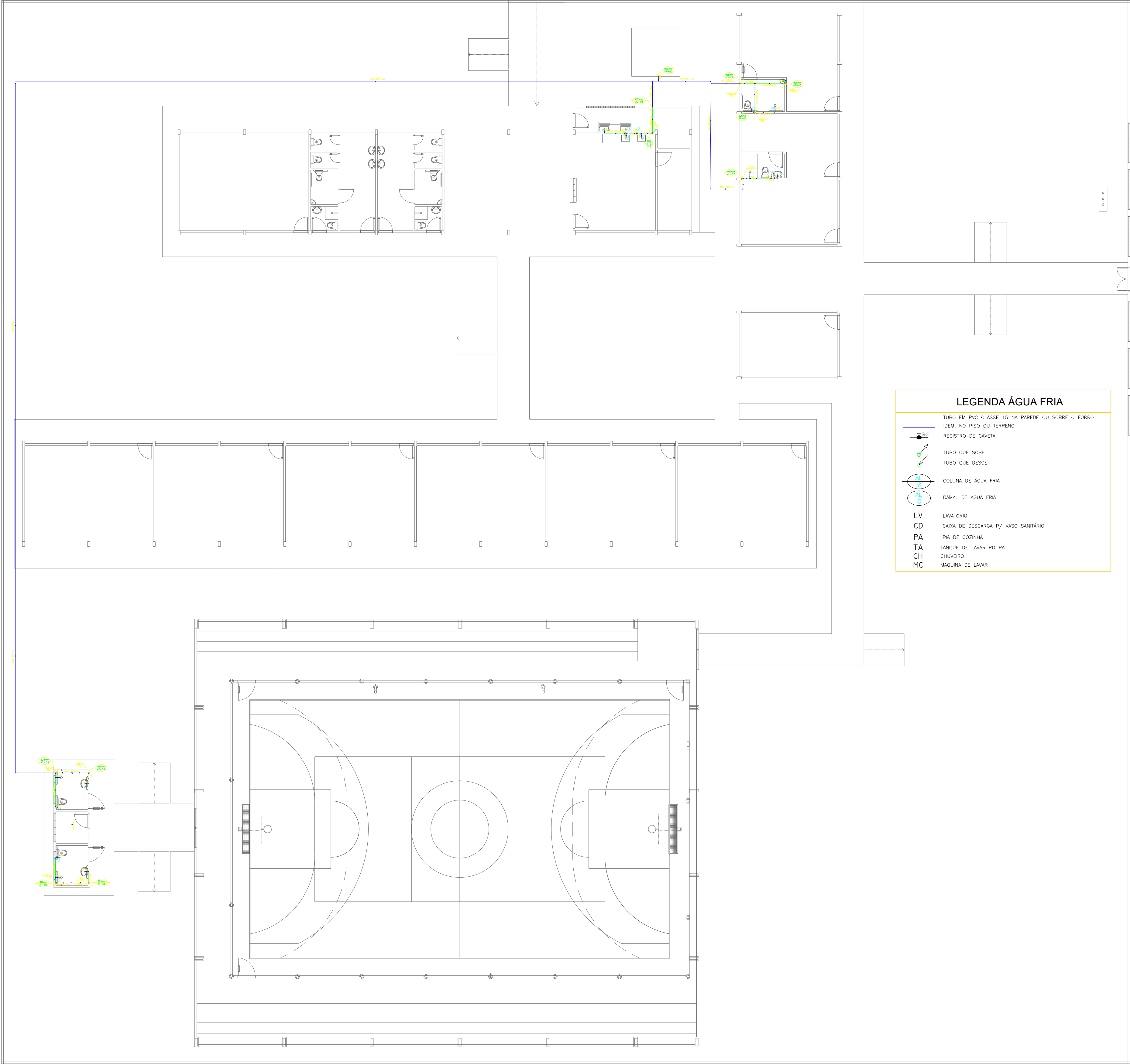
PLANTA DE AGUA FRIA ESCOLA SÃO PEDRO COMUNIDADE DE BOM JARDIM COORDENADAS: -2.559886, -54.594701 Escala 1 : 150
