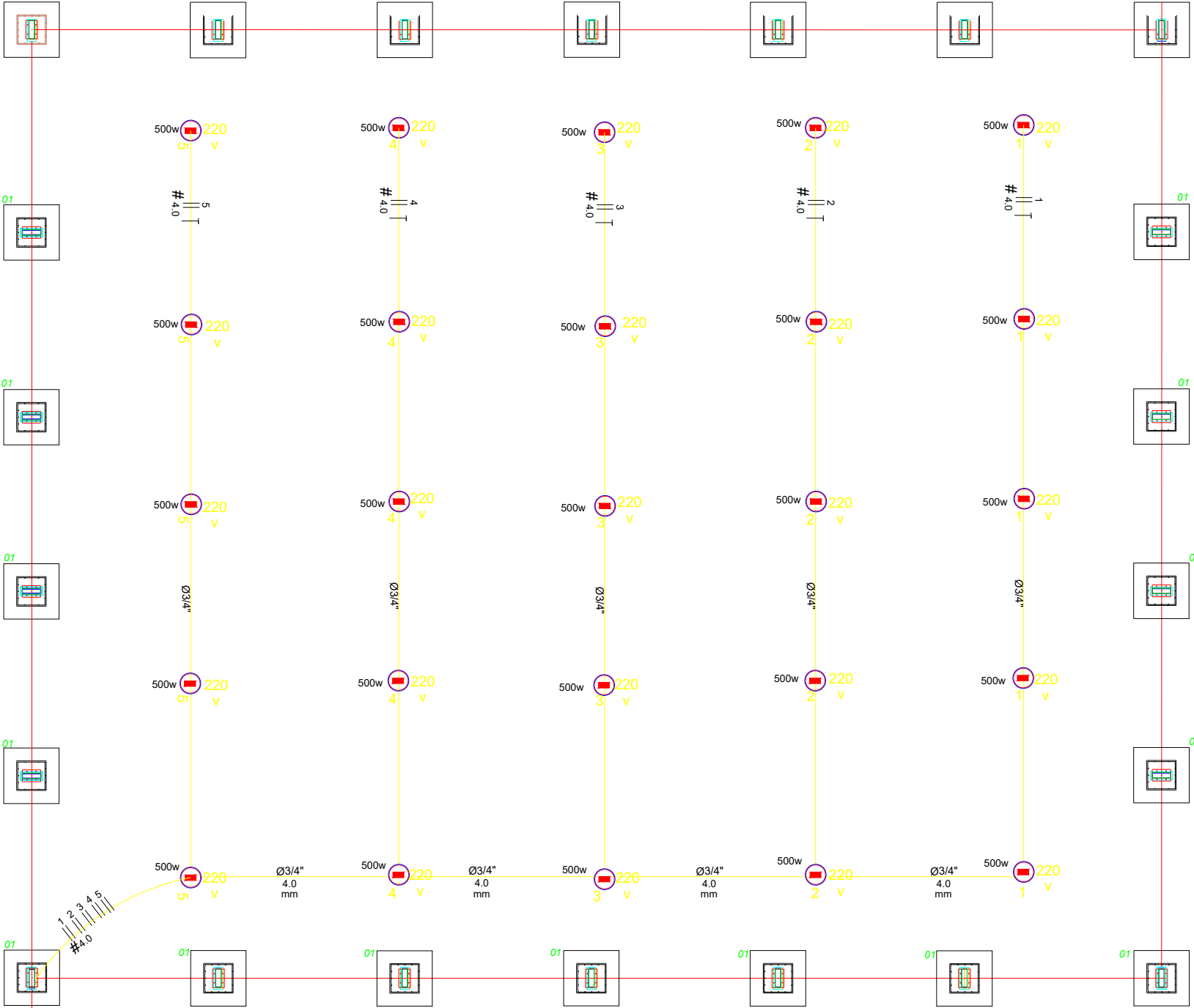
PLANTA ELÉTRICA - SUPERIOR ESCALA: 1/150
